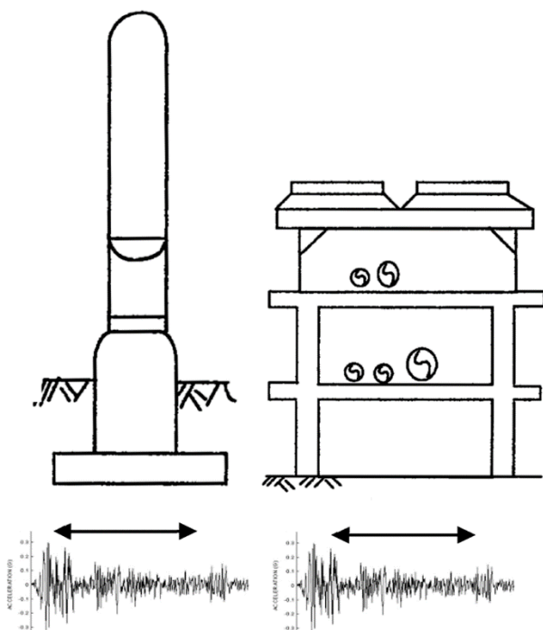
الف) هر دو سازه مجاور تحت اثر زلزله مشابه و پیش از تجربه خرابی‌ها
