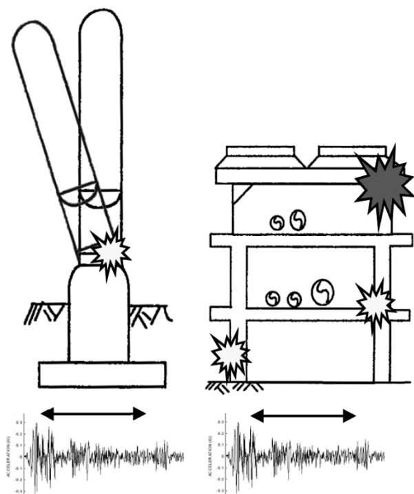
ب) هر دو سازه مجاور تحت اثر زلزله مشابه و پس از خرابی‌های درون‌سازه‌ای و بین‌سازه‌ای
