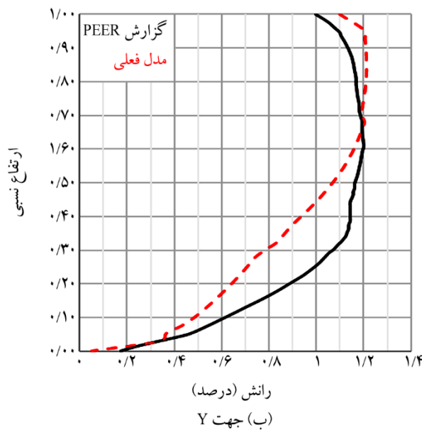
شکل (۱۰): مقایسه مقادیر Drift تحت زلزله لوما پرتا در گزارش PEER و مدل مورد نظر.
