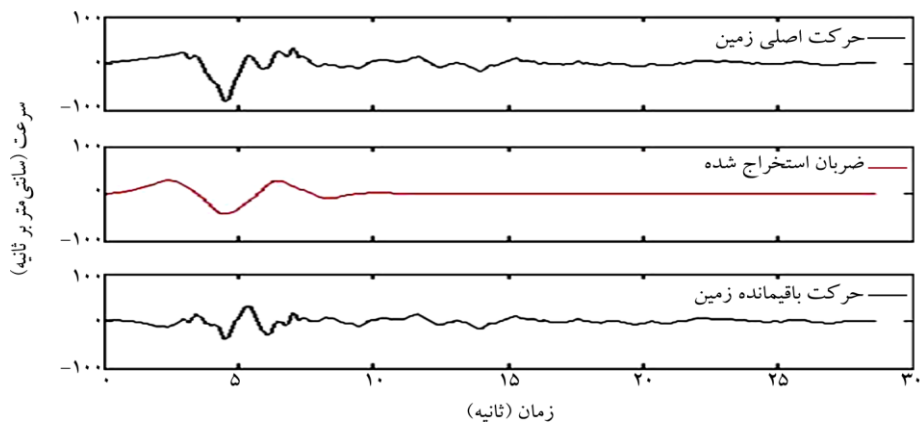
شکل (۱۴): نمودار تاریخچه زمانی سرعت برای زلزله کیپ مندوسینو.
