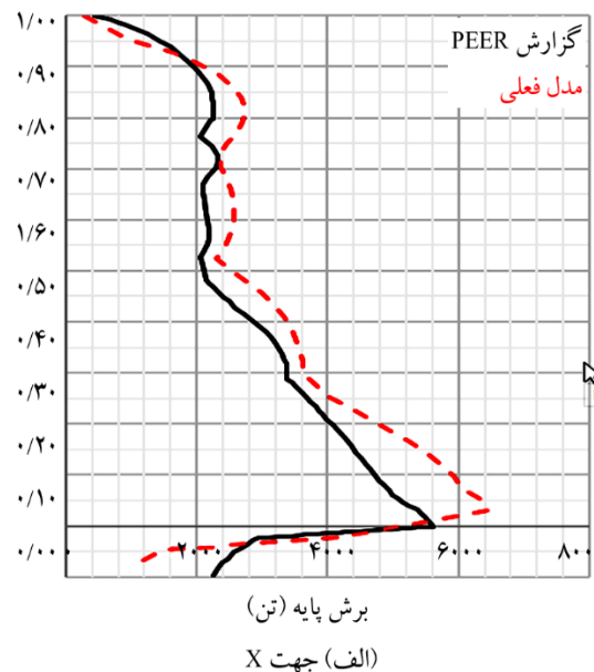
شکل (۱۱): مقایسه مقادیر برش طبقات تحت زلزله لوما پرتا در گزارش PEER و مدل مورد نظر.
