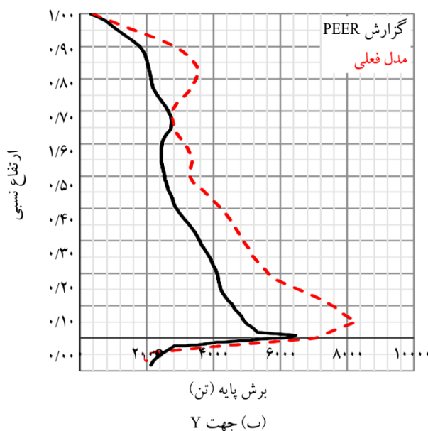
شکل (۱۱): مقایسه مقادیر برش طبقات تحت زلزله لوما پرتا در گزارش PEER و مدل مورد نظر.
