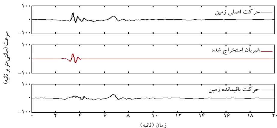
شکل (۱۲): نمودار تاریخچه زمانی سرعت برای زلزله نورتریج.
