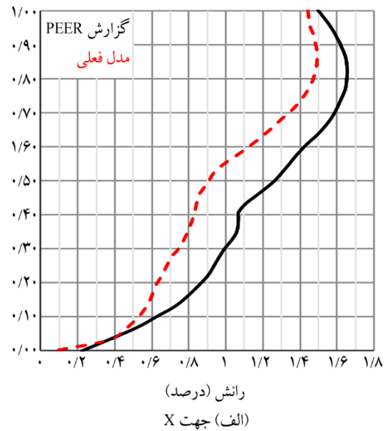
شکل (۱۰): مقایسه مقادیر Drift تحت زلزله لوما پرتا در گزارش PEER و مدل مورد نظر.
