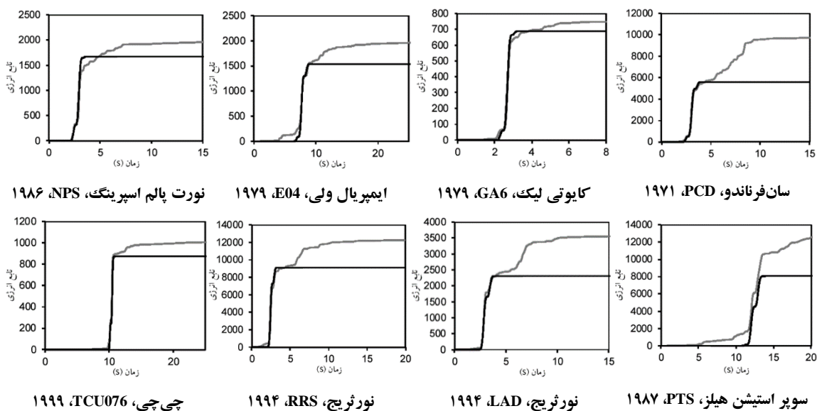
شکل (۵): تابع انرژی رکورد واقعی و پالس شبیه‌سازی شده.
