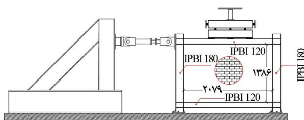
شکل (۱): پیکربندی آزمایشگاهی نمونه VL (تمامی ابعاد به میلی‌متر می‌باشد).
