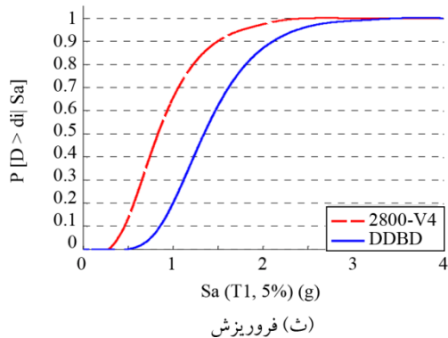
شکل (۱۲): منحنی‌های شکنندگی قاب ۱۱ طبقه در سطوح خرابی مختلف.
