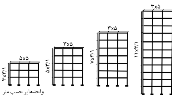
شکل (۱): پارامترهای هندسی قاب های مدل سازی شده.
