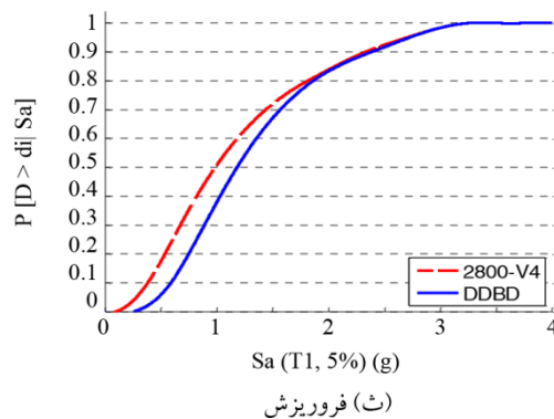
شکل (۱۱): منحنی‌های شکنندگی قاب ۵ طبقه در سطوح خرابی مختلف.
