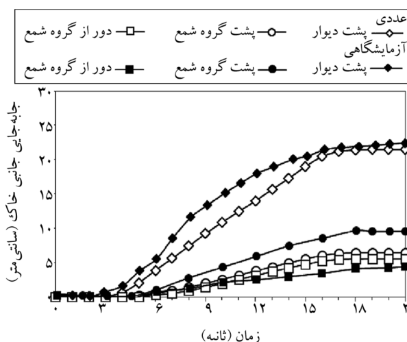
شکل (۱۰): تاریخچه زمانی جابه‌جایی جانبی سطحی در نقاط مختلف.
