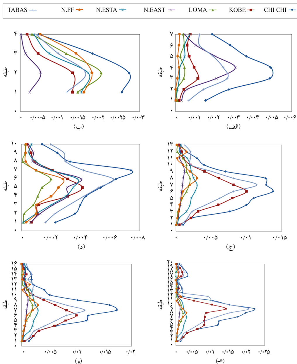
شکل (۶): نمودار میانگین دوران پلاستیک بر حسب رادیان، تحت اثر زلزله منفرد ساختمان (الف) ۴ طبقه، (ب) ۷ طبقه، (ج) ۱۰ طبقه، (د) ۱۳ طبقه، (ه) ۱۶ طبقه، (و) ۲۰ طبقه.
