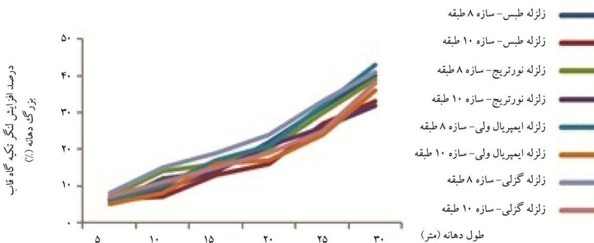
شکل (۵): مقادیر لنگر تکیه گاه قاب بزرگ دهانه نسبت به طول دهانه در اثر زلزله های مختلف.
