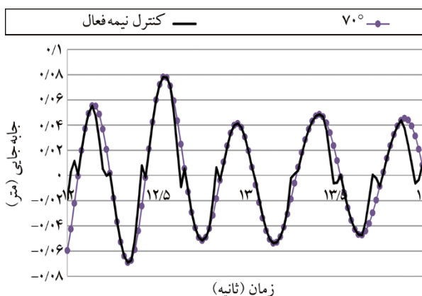
شکل (۵): نمودار تاریخچه زمانی جابه‌جایی بام تحت اثر زلزله کوبه تحت کنترل نیمه فعال و پره با زاویه ۷۰ درجه.
