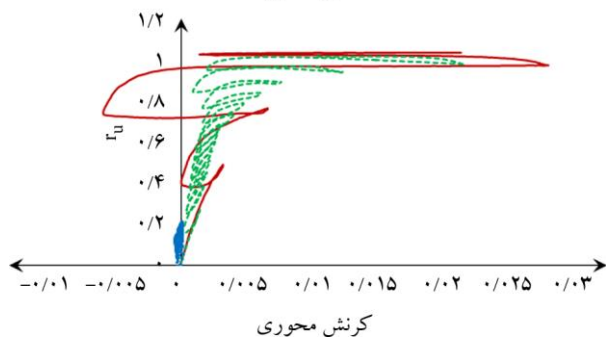
شکل (۱۱): تأثیر CSR بر تغییرات \tau_u بر حسب کرنش محوری در M.
