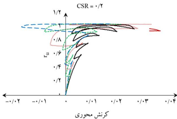
شکل (۱۲): تأثیر میزان ریزدانه در CSR = 0.2 بر تغییرات \tau_u بر حسب کرنش محوری.
