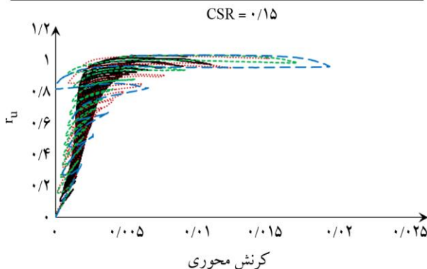
شکل (۱۳): تأثیر میزان ریزدانه در CSR = 0.15 بر تغییرات \tau_u بر حسب کرنش محوری.
