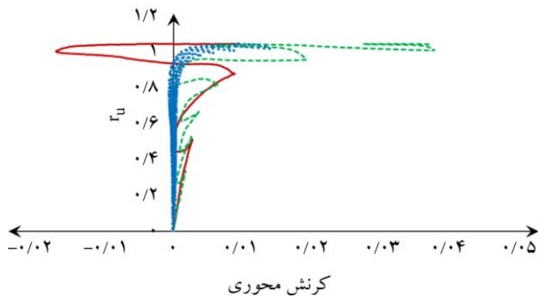
شکل (۱۰): تأثیر CSR بر تغییرات \tau_u بر حسب کرنش محوری در S7M3.
