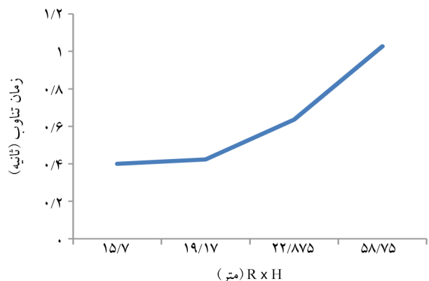
شکل (۹): تغییرات زمان تناوب مخازن مورد مطالعه با حاصل ضرب ارتفاع سازه در شعاع مخزن (متر).
